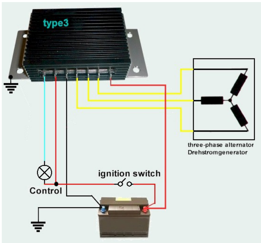
Abbildung 2 Schematischer Anschlussplan
