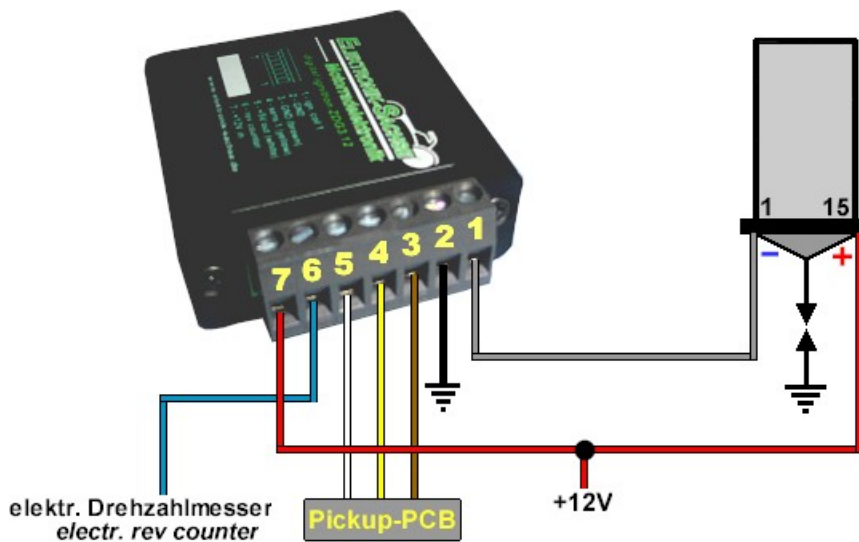
Abbildung 4 Anschlußschema
