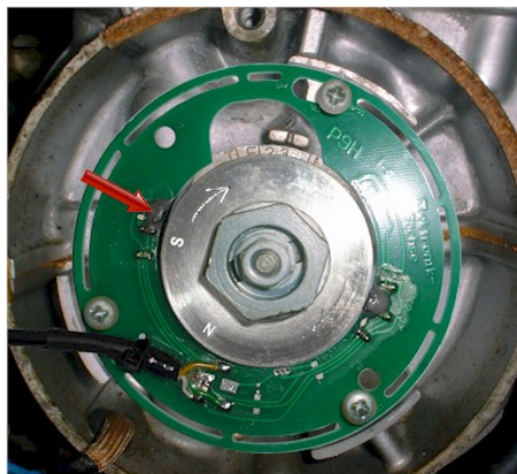
Abbildung 7.a Auf diesem Sensor wird die Grundeinstellung gemacht.
