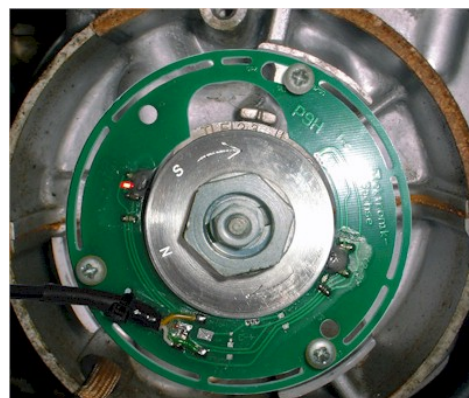
Abbildung 7.b Die LED geht an, wenn der S-Magnet am Sensor vorbeiläuft.
