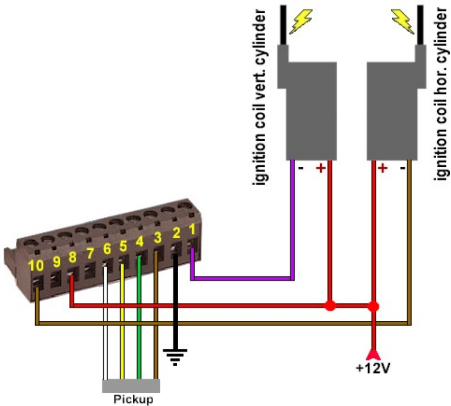
Abbildung 3 Anschlußschema
