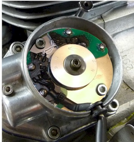
Abbildung 2.e Fertige Montage des Pickups
