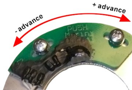
Abbildung 7.b Feineinstellung des Versatzes der Frühzündung zwischen den beiden Zylindern.
