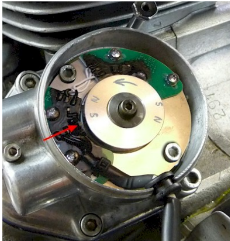
Abbildung 7.a Dieser Sensor wird für die Grundeinstellung benutzt.
