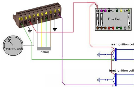
Abbildung 3 Anschlußschema
