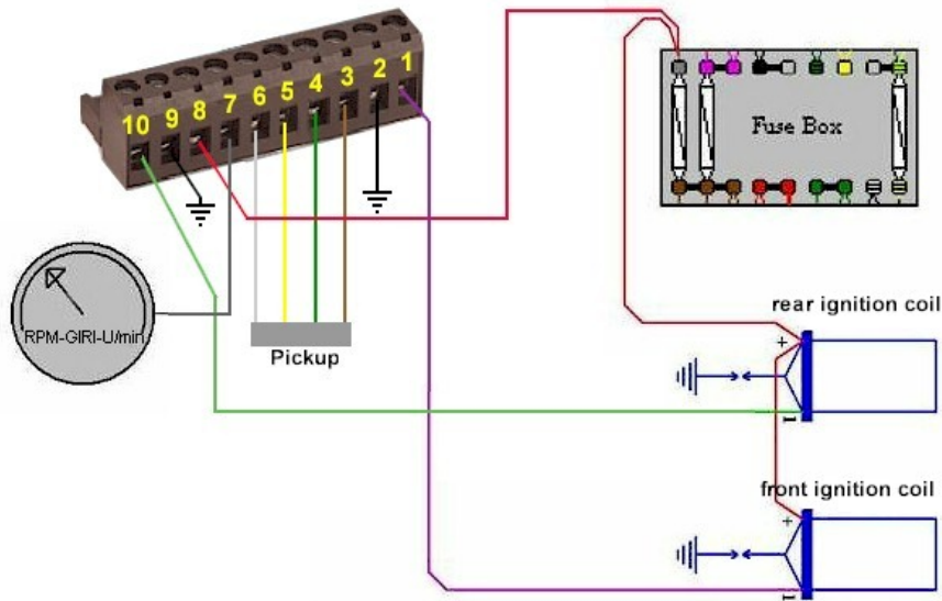
Anschlussschema
