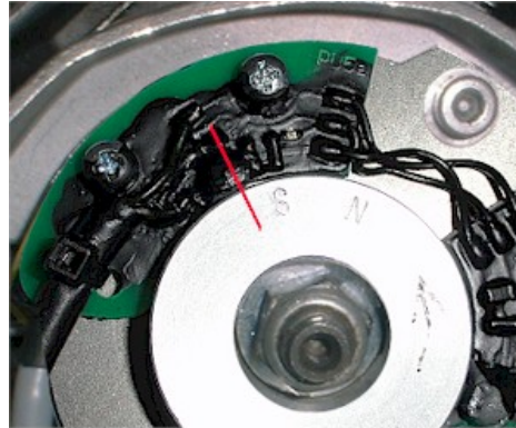
Abbildung 6.b Dieser Sensor wird für die Grundeinstellung benutzt.
