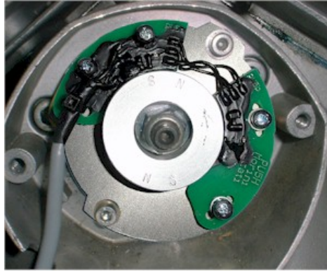
Abbildung 2.a Montage von Pickup
