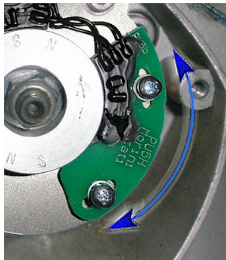
Abbildung 6.d Feineinstellung des Versatzes der Frühzündung zwischen den beiden Zylindern.
