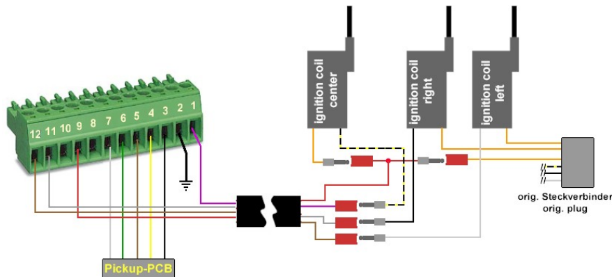
Elektrischer Anschluss der Zündung
