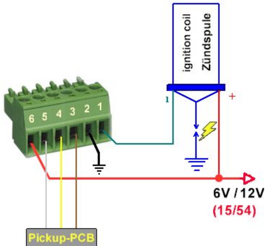
Anschlusschema
