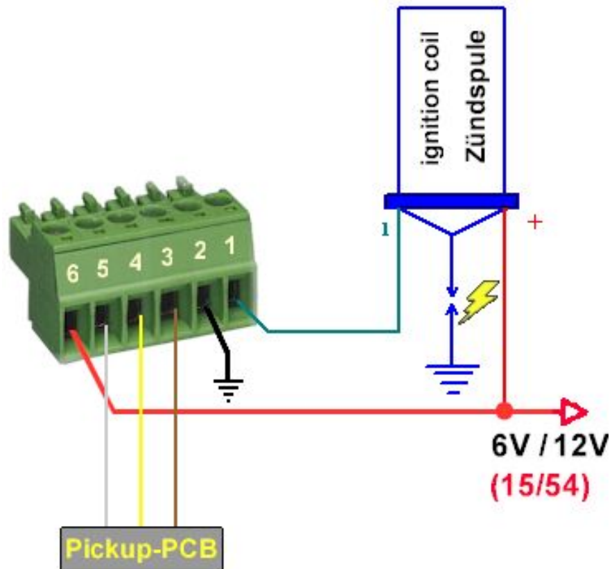
Anschlusschema
