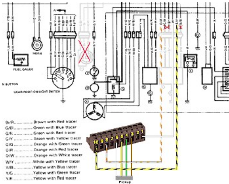
Anschlussschema
