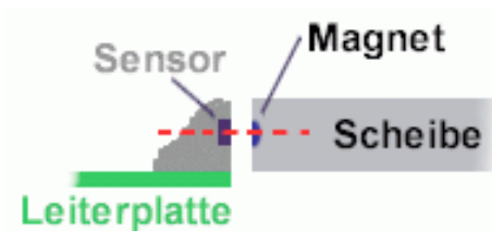
Abbildung 5 Korrekte Ausrichtung von Magnetrings und Sensor.
