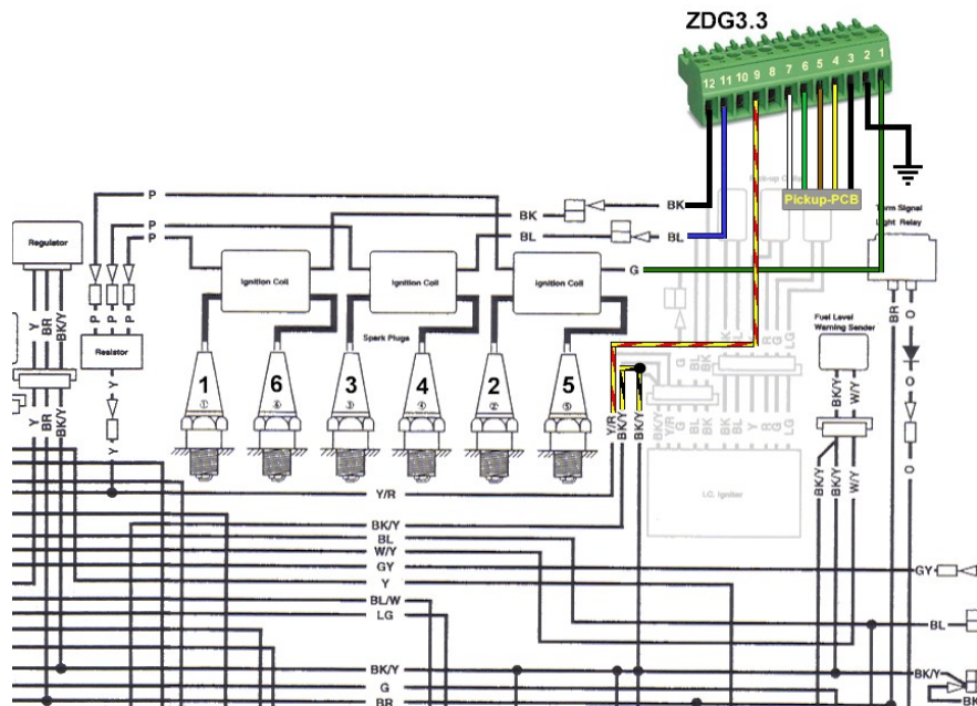
Anschlussdiagramm
