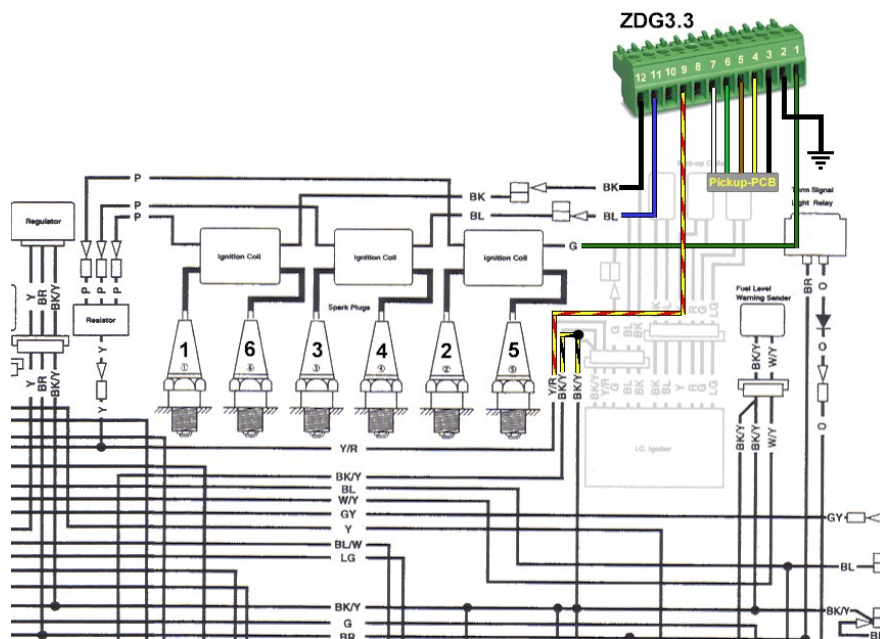
Abbildung 3 Anschlußschema
