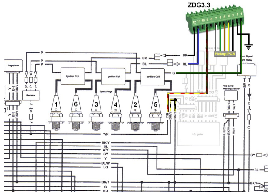
Abbildung 3 Anschlußschema
