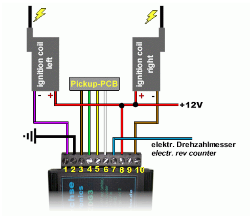
Elektrischer Anschluss
