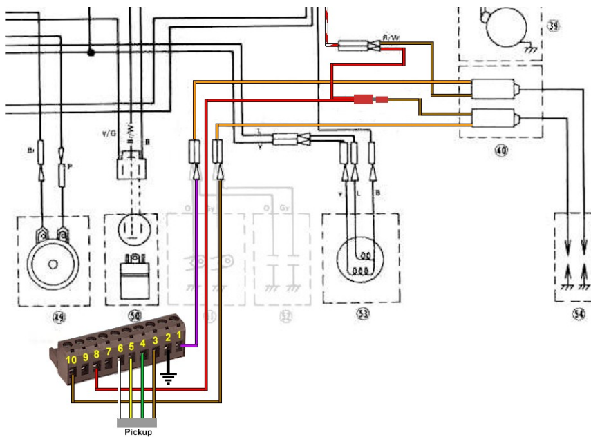
Anschluss im originalen Schaltbild
