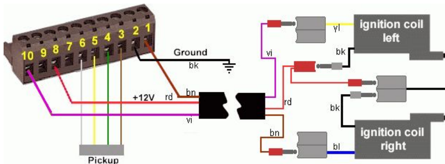
Elektrischer Anschluss der Zündung
