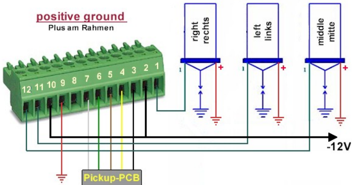
Anschlussschema der Zündung mit Plus am Rahmen
