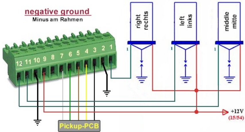
Anschlussschema der Zündung mit Minus am Rahmen
