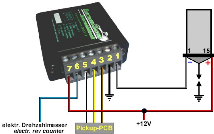
Elektrischer Anschluss der Zündung
