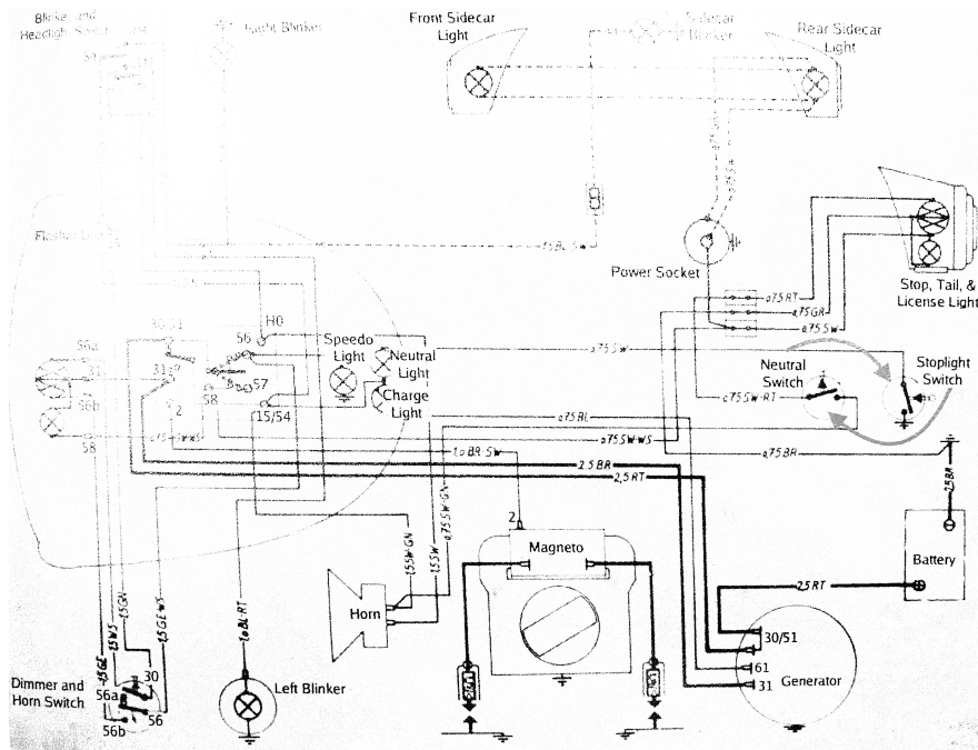
Abbildung 2 Originalschaltplan von der R69S.
