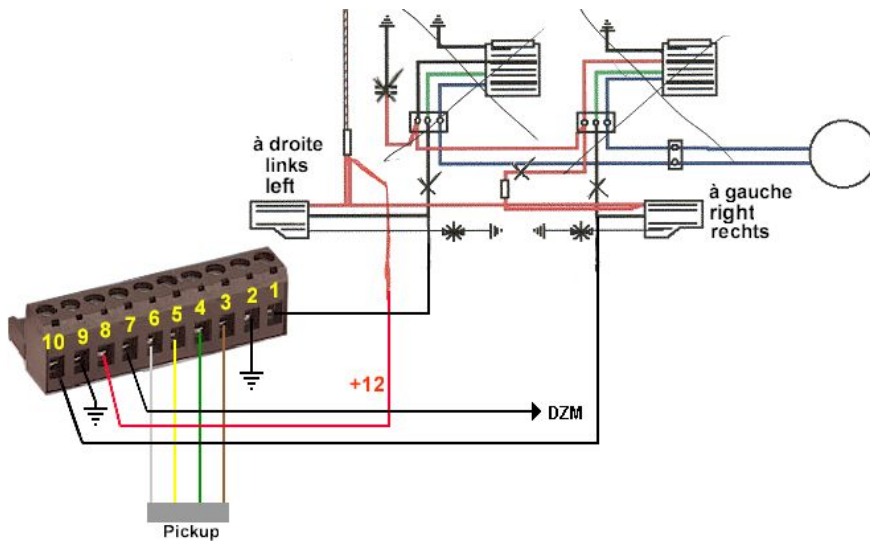
Anschlussschema der Zündung bei Motoplatt-Ersatz
