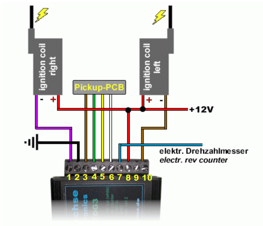
Anschlussschema der Zündung bei Kontakt-Ersatz
