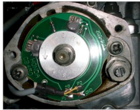
Pickup_Leiterplatte CB450
