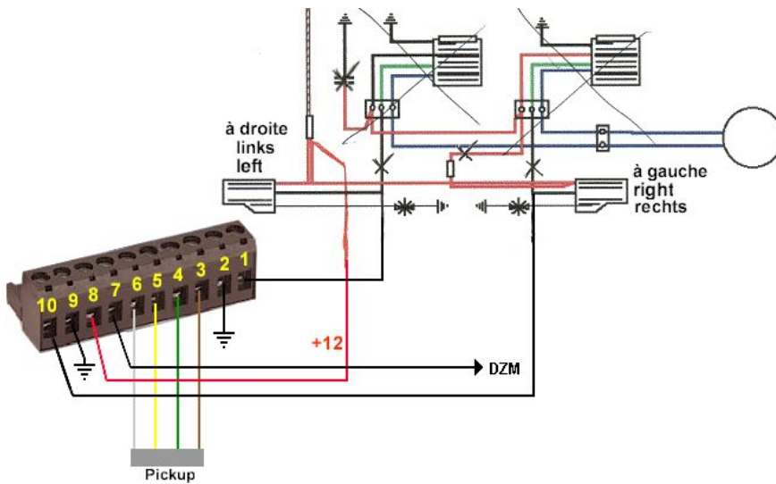
Anschlussschema der Zündung bei Motoplat-Ersatz
