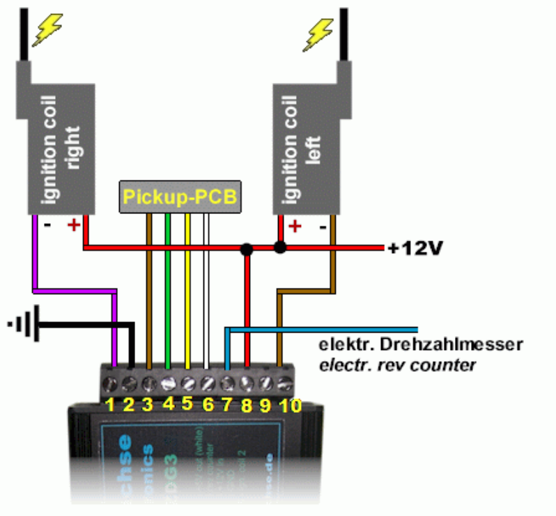
Anschlusschema der Zündung bei Motoplat-Ersatz
