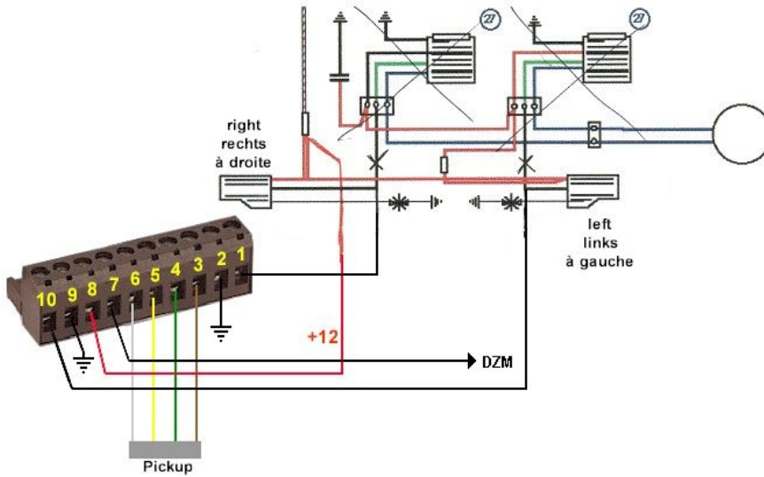
Anschlusschema der Zündung bei Kontakt-Ersatz
