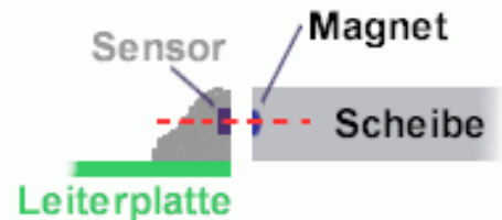
Abbildung 3 Korrekte Ausrichtung von Magnetring und Sensor.
