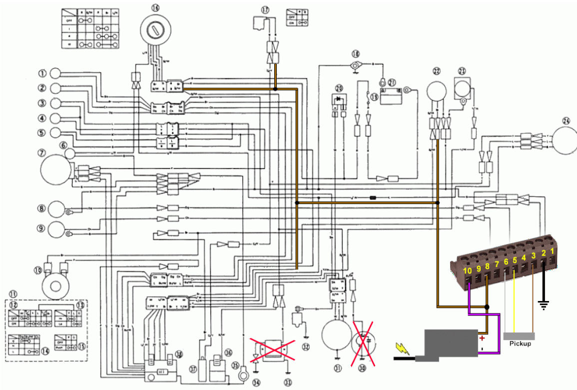
Anschlussschema
