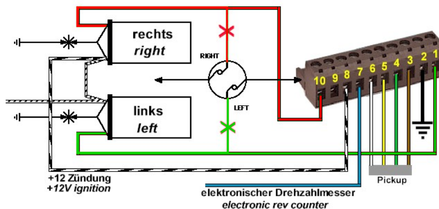
Abbildung 2 Anschlußschema der Zündung bei Kontaktersatz
