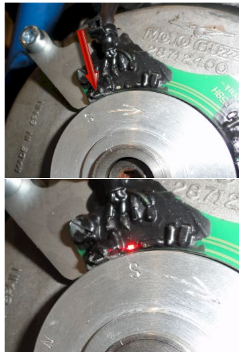
Abbildung 5 Ausrichten des Magnetringes so daß die LED gerade an- bzw. ausgeht.
