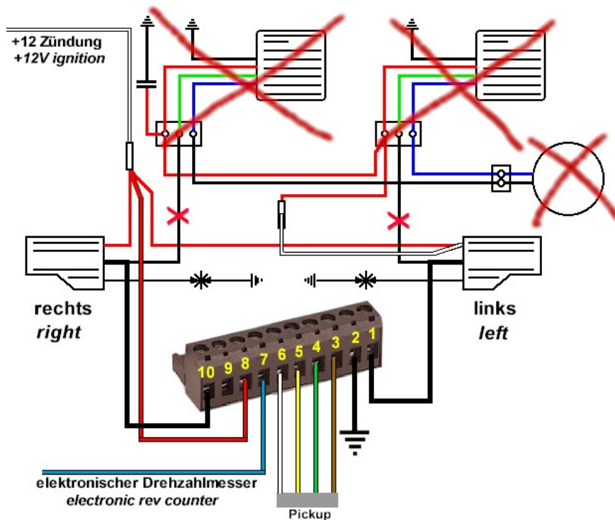
Abbildung 2 Anschlußschema der Zündung bei Motoplatt-Ersatz
