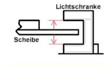
Abbildung 2 Ausrichtung von Sektorscheibe und Lichtschranke.
