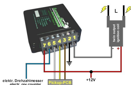
Elektrischer Anschluss der Zündung mit einer 12 V-Doppelzündspule.
