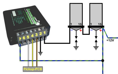
Elektrischer Anschluss der Zündung mit zwei 6 V-Zündspulen in Reihe.
