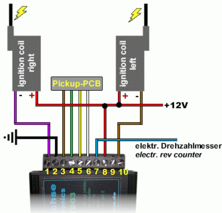
Elektrischer Anschluss der Zündung mit zwei 12 V-Zündspulen.
