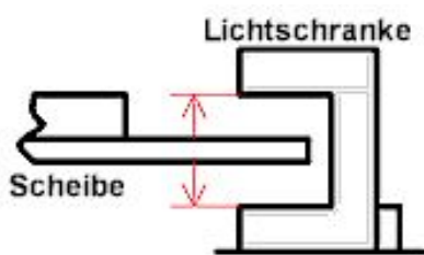
Abbildung 2 Ausrichtung von Sektorscheibe und Lichtschranke.
