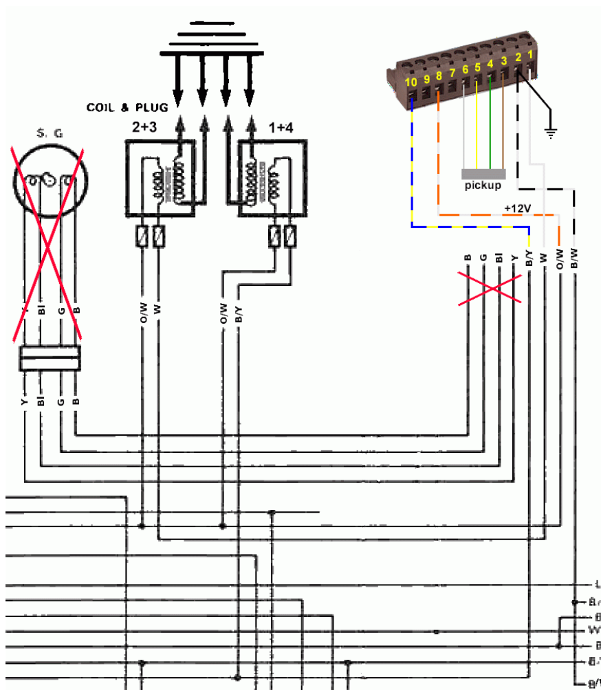
Komplettes Schaltbild
