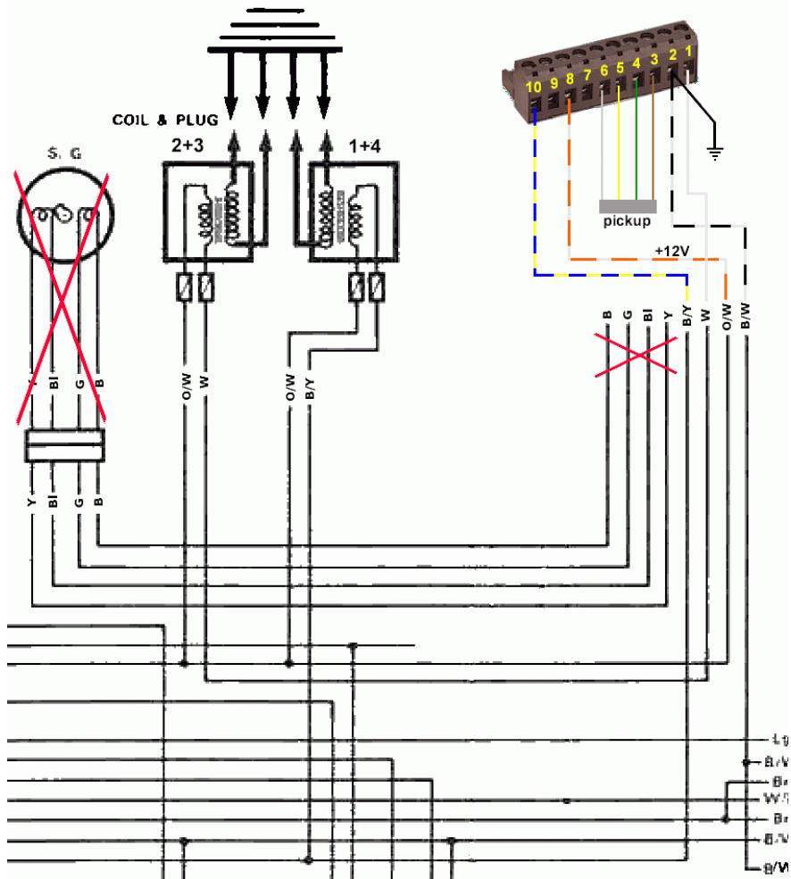
Anschlusschema
