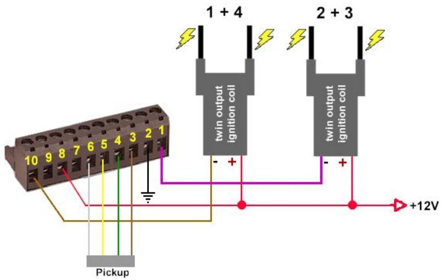
Anschlusschema
