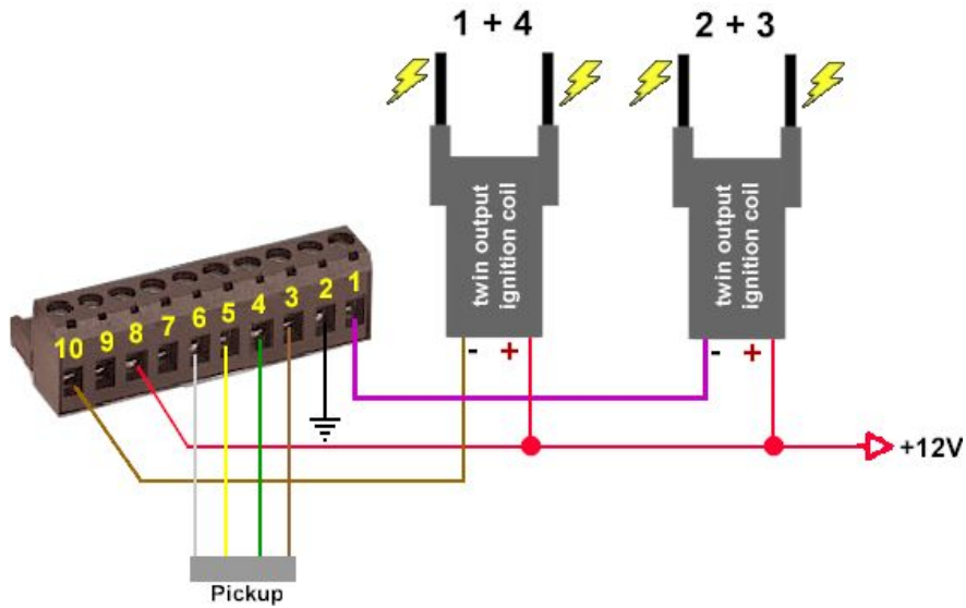
Anschlusschema
