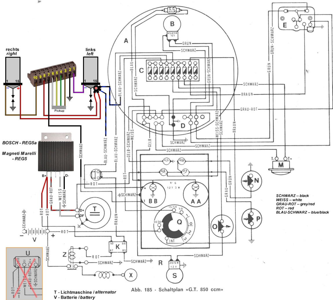
Anschluss im Stromlaufplan
