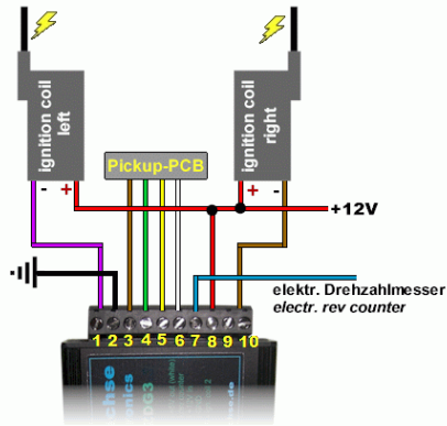
Elektrischer Anschluss der Zündung
