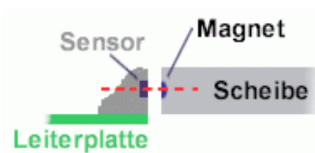
Abbildung 2 Korrekte Ausrichtung von Magnetring und Sensor.
