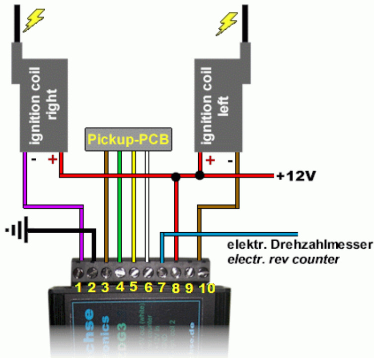
Elektrischer Anschluss der Zündung
