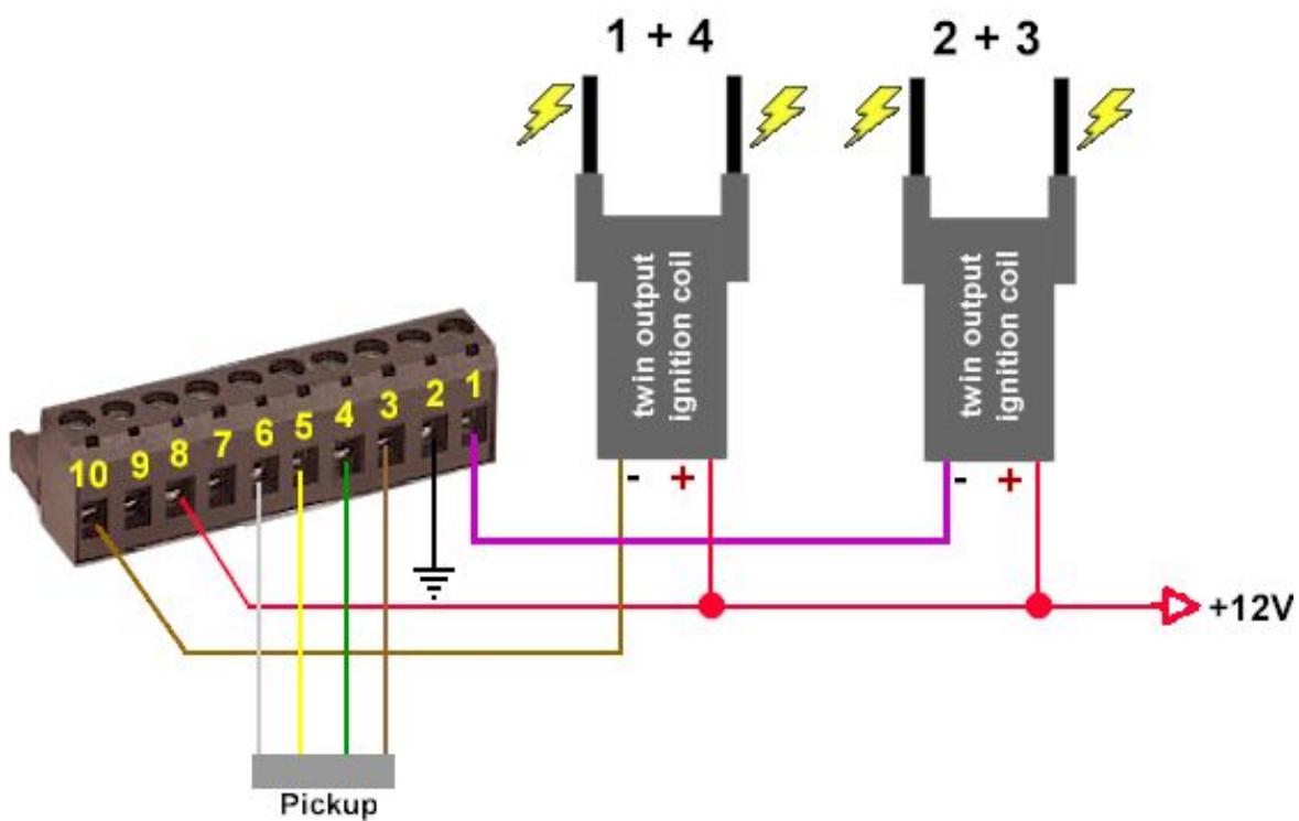
Anschlusschema
