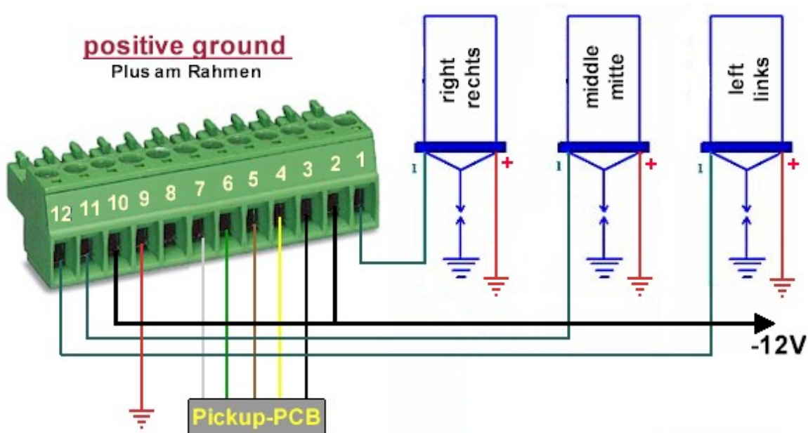
Anschlusschema der Zündung mit Plus am Rahmen
