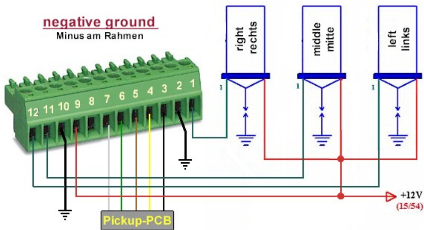
Anschlusschema der Zündung mit Minus am Rahmen
