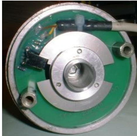
Abbildung 2.d Fertig eingebaute Zündung (ältere optische Variante ist hier abgebildet, die aktuelle nutzt Halleffectsensoren und sieht etwas anders aus).
