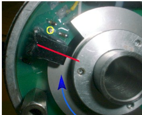
Abbildung 6 Wenn die LED auf OT ausgeht, dann ist die Zündung korrekt eingestellt. Zu beachten ist, daß diese Abbildung die ältere optische Version zeigt.
