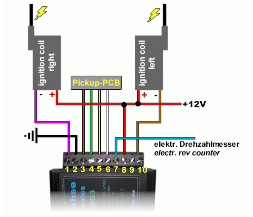
Abbildung 3 Anschlußschema
