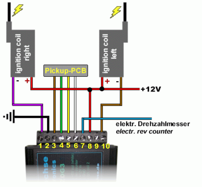
Abbildung 3 Anschlußschema
