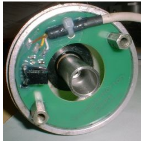
Abbildung 2 Montage des Pickups (hier abgebildet ist eine ältere Version).
