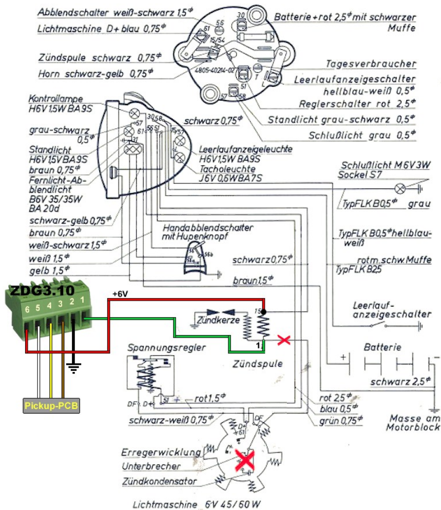
Anschluss im Stromlaufplan
