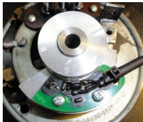
Zuletzt den Magnetring auf den Mitnehmer stecken (Pfeil nach rechts), aber die Madenschrauben noch nicht festziehen.
