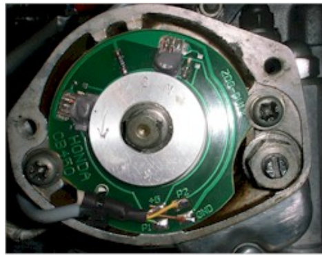
Pickup_Leiterplatte CB450
