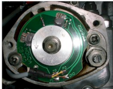
Pickup_Leiterplatte CB450
