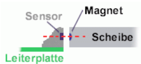
Abbildung 8 Korrekte Ausrichtung von Magnetring und Sensor.
