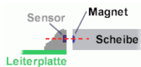
Abbildung 8 Korrekte Ausrichtung von Magnetring und Sensor.
