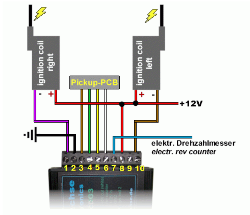
Abbildung 6 Anschlußschema
