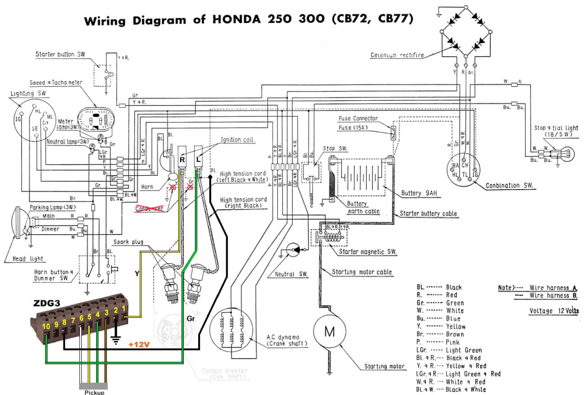
Abbildung 5 Anschluß im Stromlaufplan
