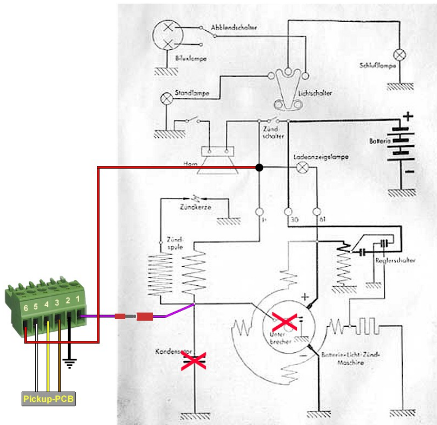
Anschluss im Stromlaufplan
