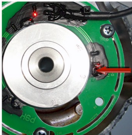
Abbildung 6 Dieser Sensor wird für die Grundeinstellung verwendet.
