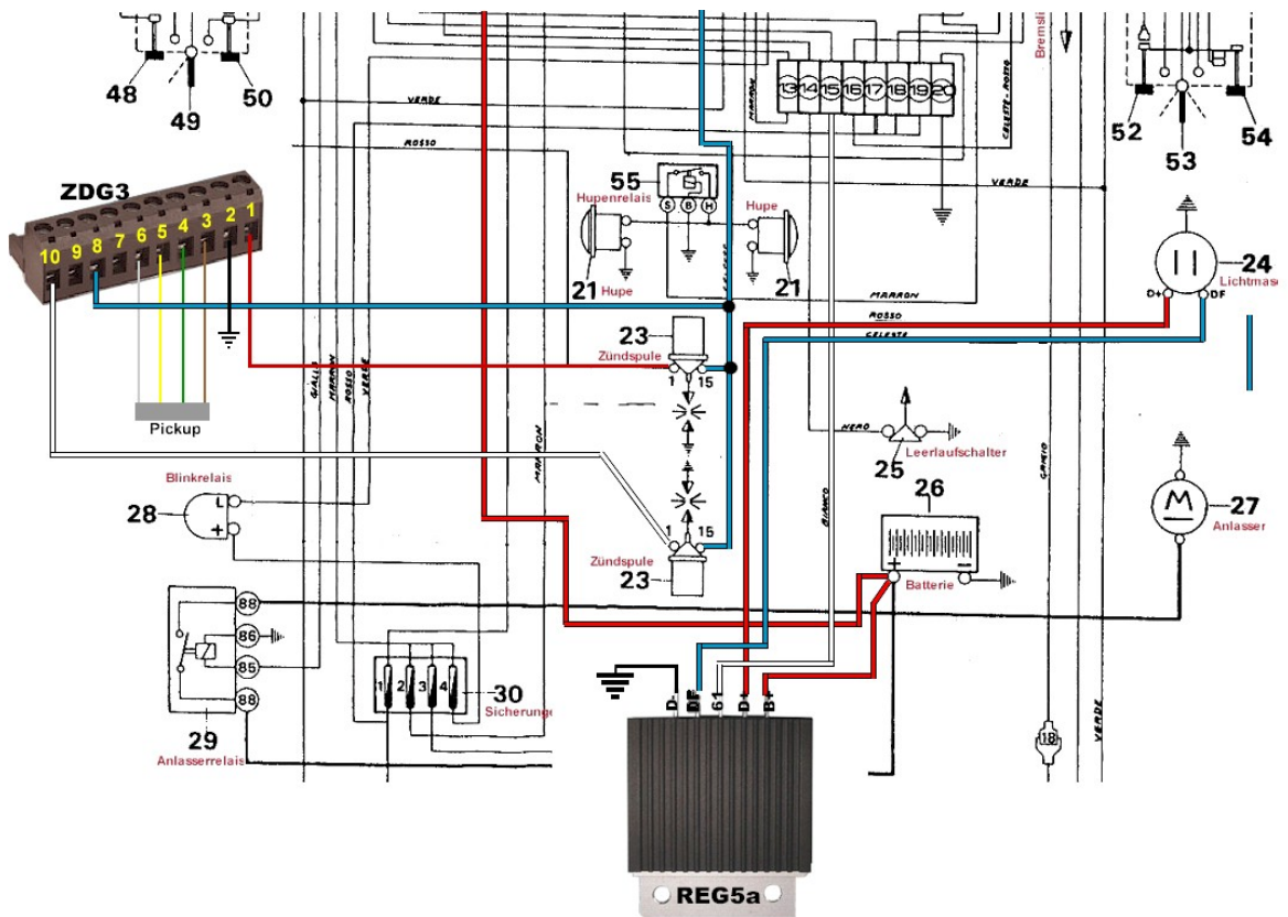
Abbildung 4 Anschlußdiagramm (mit Regler REG5a)
