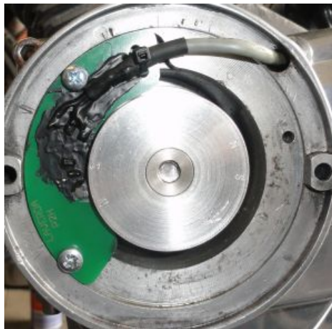
Abbildung 2 Montage des Magnetringes.
