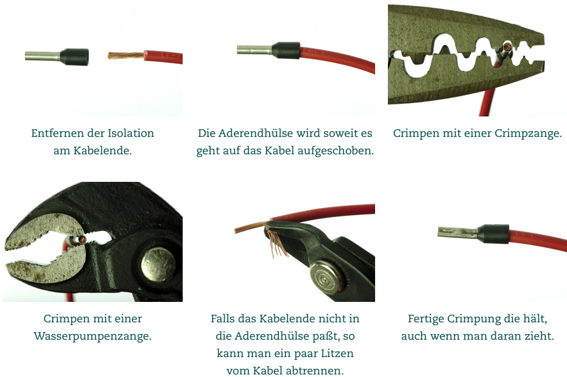
Abbildung 5 Crimpen der Aderendhülsen
