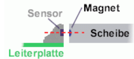
Abbildung 6 Korrekte Ausrichtung von Magnetring und Sensor.
