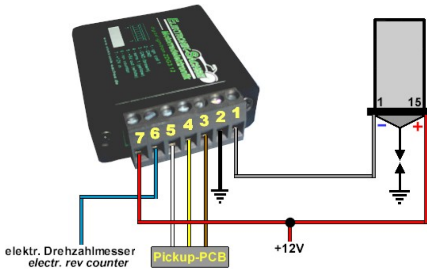
Anschlußschema
