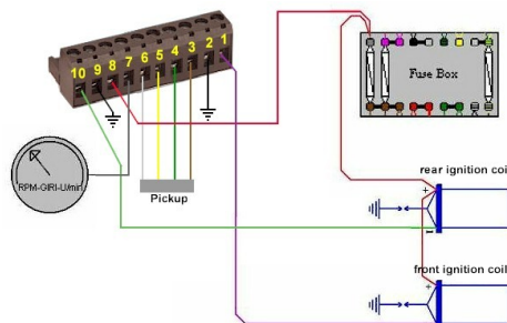
Abbildung 3 Anschlußschema
