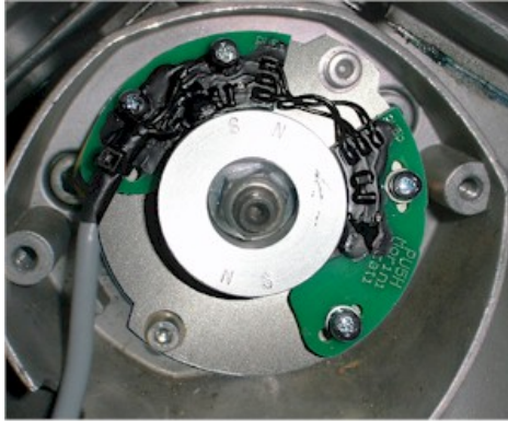
Abbildung 2 Montage von Pickup
