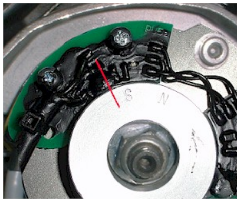
Abbildung 6 Dieser Sensor wird für die Grundeinstellung benutzt.
