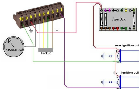
Abbildung 3 Anschlußschema
