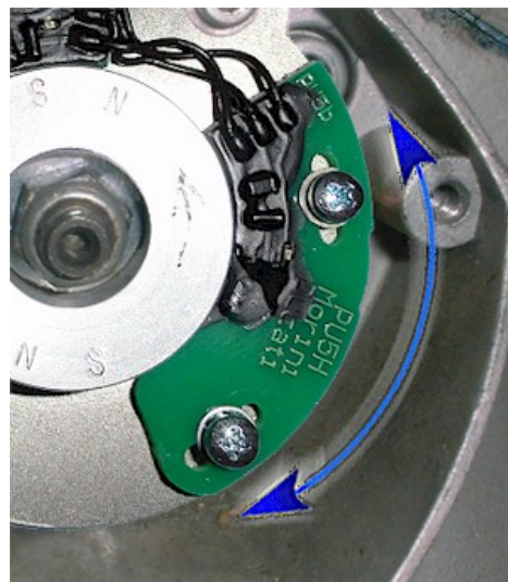
Abbildung 6 Feineinstellung des Versatzes der Frühzündung zwischen den beiden Zylindern.
