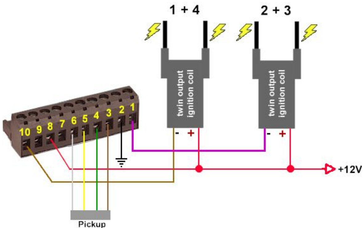
Anschlussschema
