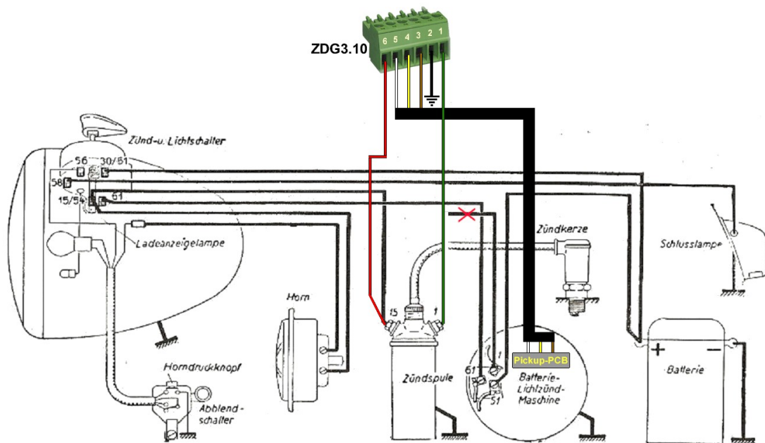
Abbildung 3 Anschlussschema
