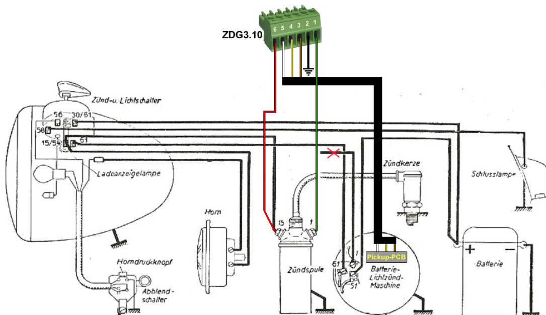
Abbildung 3 Anschlussschema
