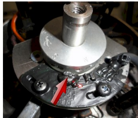
Abbildung 5 Dieser Sensor wird für die Grundeinstellung verwendet.
