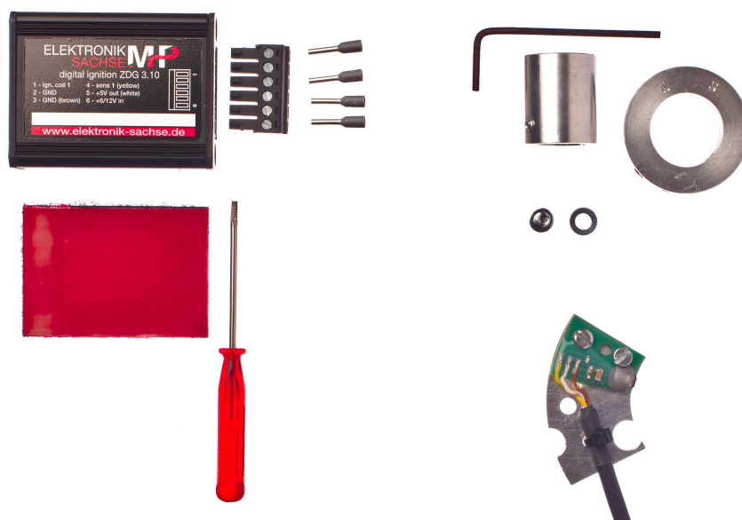
Abbildung 1 Lieferumfang
