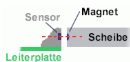
Abbildung 5 Korrekte Ausrichtung von Magnetring und Sensor.
