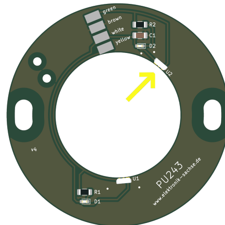
Abbildung 7 Dieser Sensor wird für die Grundeinstellung verwendet.
