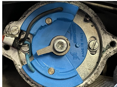
Abbildung 2 Entfernen der originalen Komponenten. Guzzi-Pickup.
