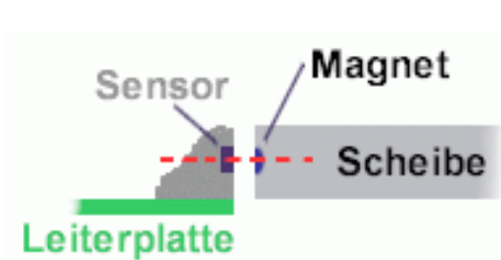
Abbildung 6 Korrekte Ausrichtung von Magnetring und Sensor.
