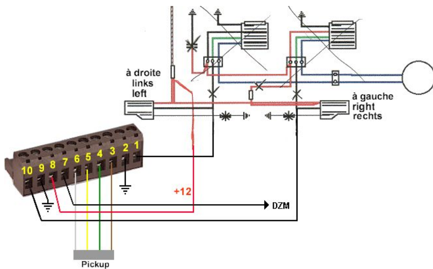
Abbildung 4 Verbindungen im Originalschaltplan.
