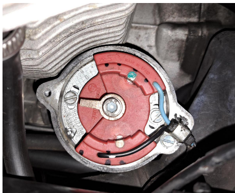
Abbildung 2 Entfernen der originalen Komponenten. Motoplat-Pickup.
