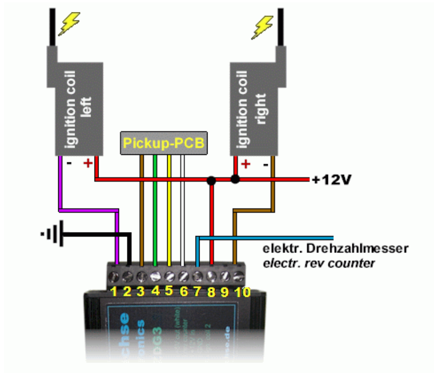
Abbildung 3 Anschlußdiagramm
