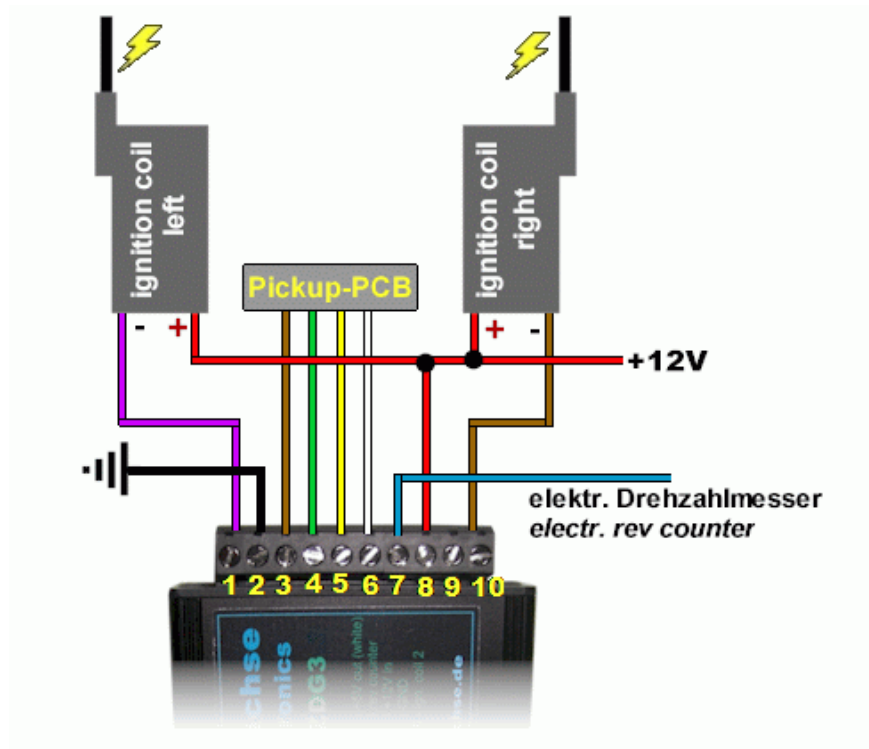
Abbildung 8 Anschlussschema der Zündung bei Kontaktersatz.
