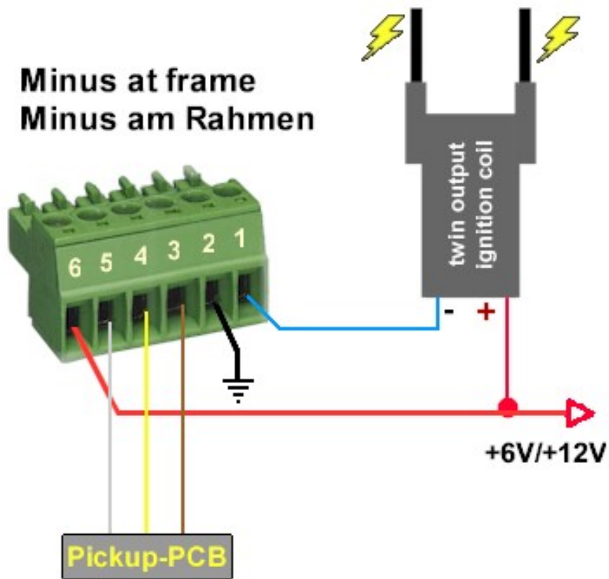
Anschlusschema
