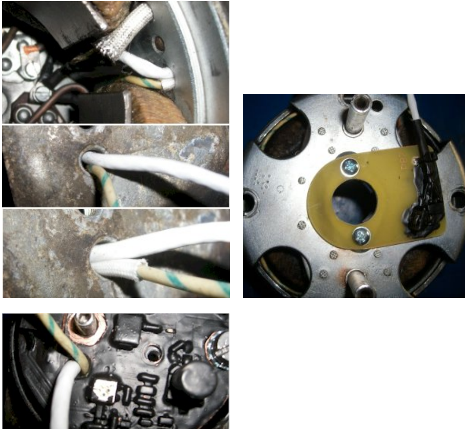
Kabelführung durch die Reglergrundplatte mit dem Lichtmaschinenregler RegKS (nicht mehr lieferbar)
