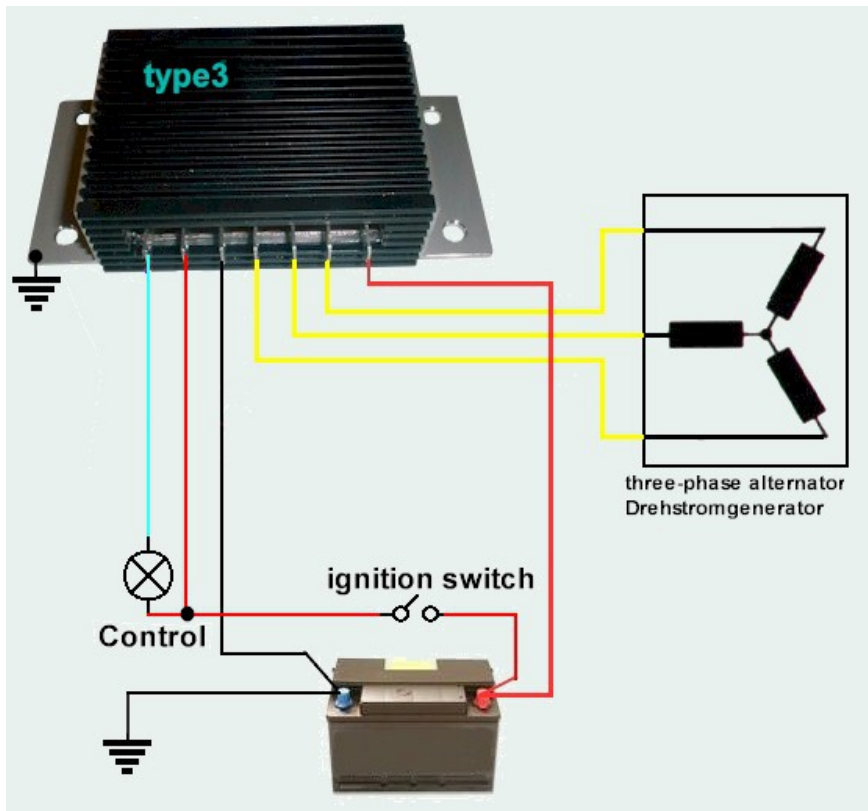
Abbildung 2 Schematischer Anschlussplan
